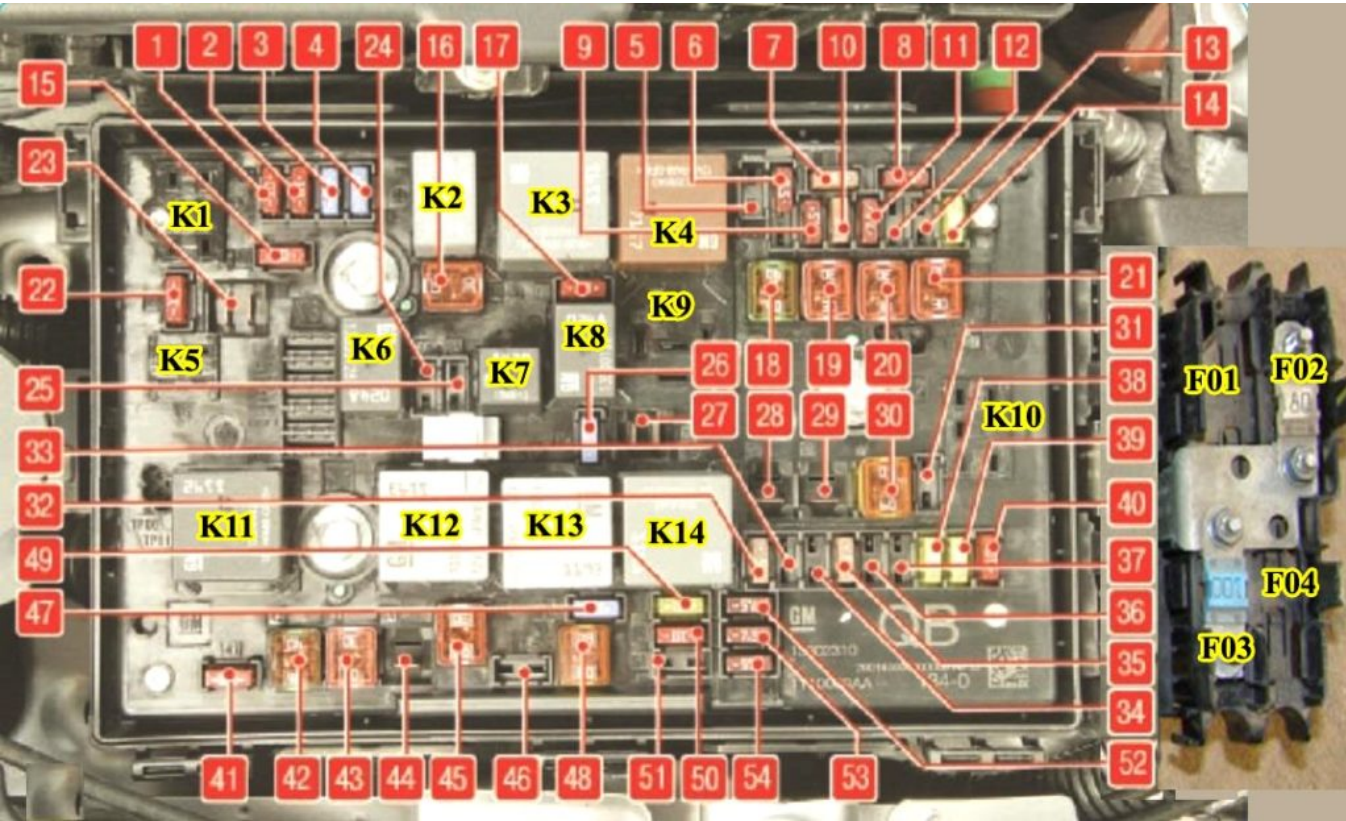
Beschreibung der Sicherungen
